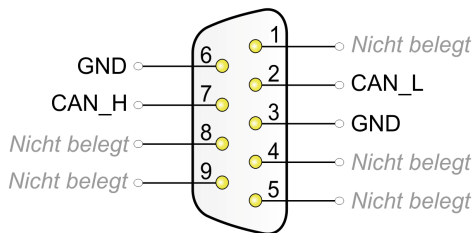
Abbildung 1: Anschlussbelegung High-Speed-CAN
