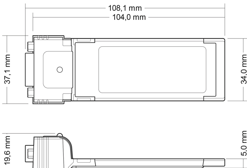
Abbildung 11: Seitenansicht und Draufsicht PCAN-ExpressCard 34
